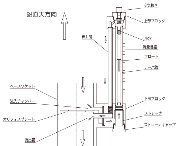
図1 測定原理図
