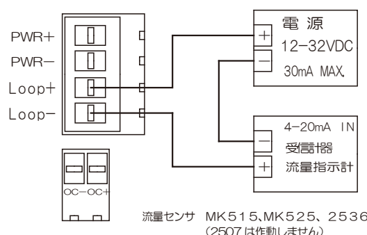
結線図11. 4-20mADC 出力 (2線式)
