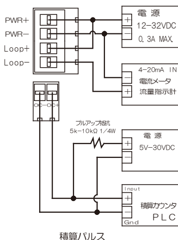
結線図15. 4-20mADC、O.C. パルス、リレー接点出力
