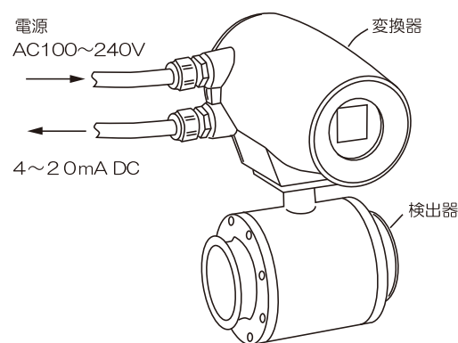
図2 構成図
