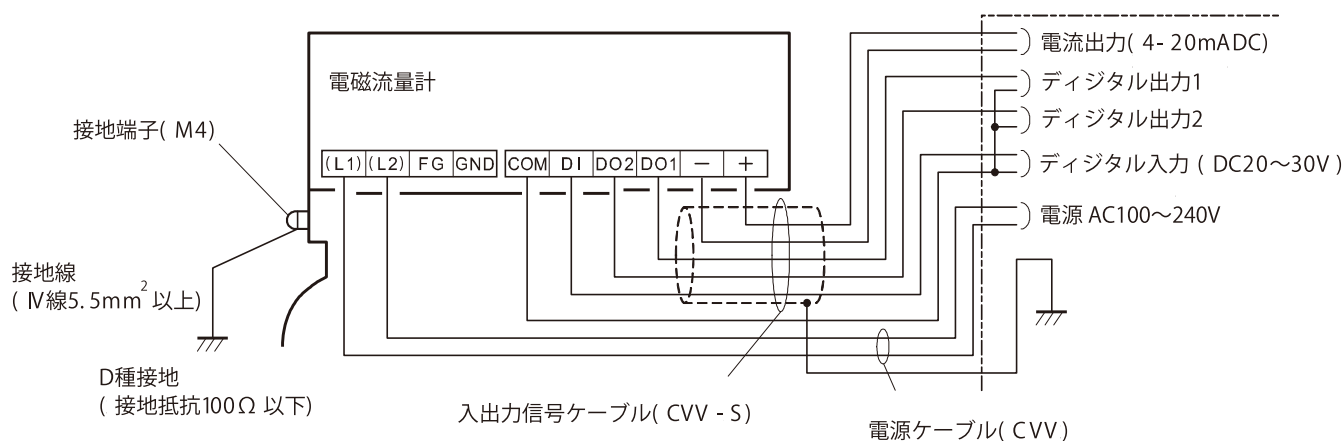
図 4 配線接続図
