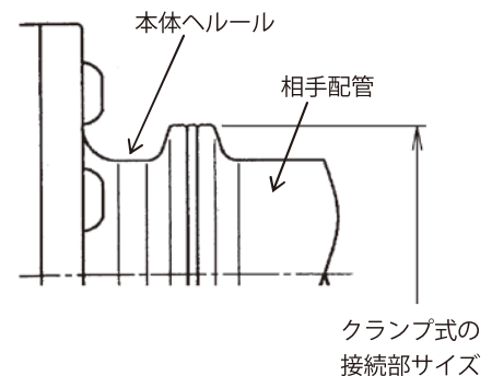
図 5 相手配管と接続する部分の位置
