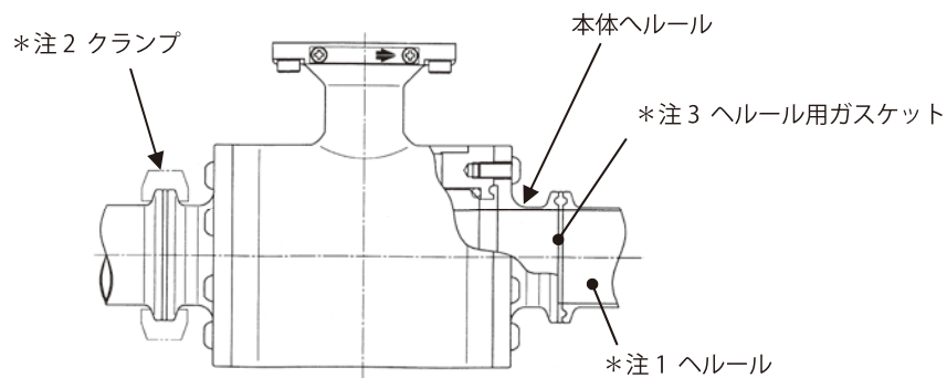
図 6 クランプ式配管接続部品名称
