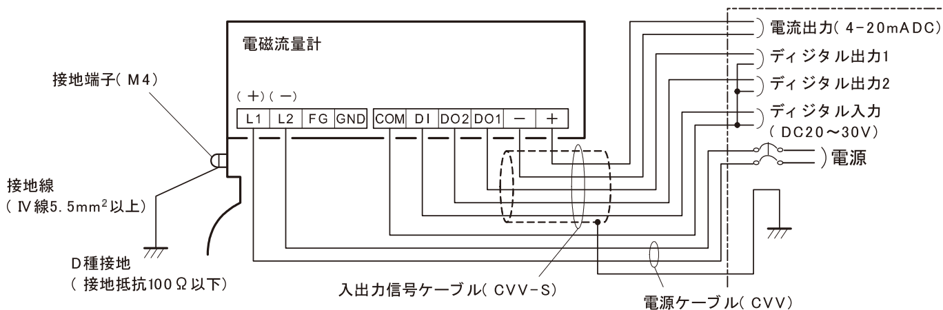
図4 配線接続図
