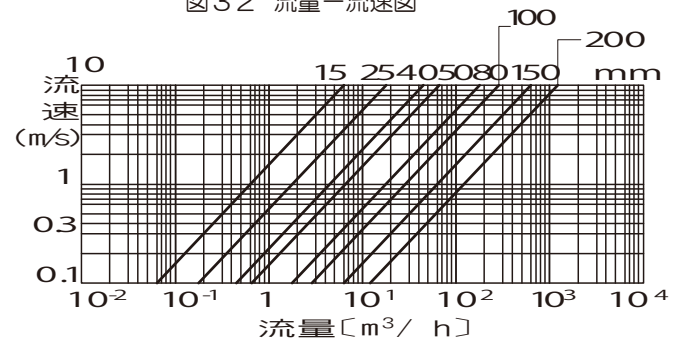
図32 流量一流速図
