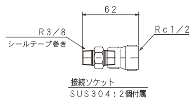
口径：1/2B サイズの構造
