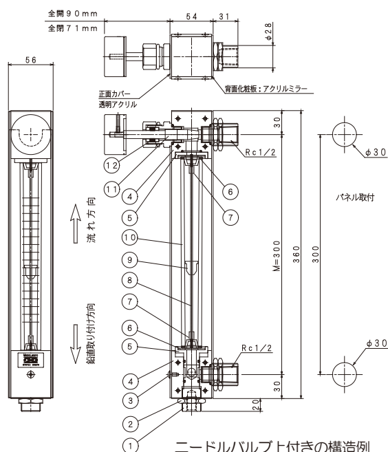
ニードルバルブ上付きの構造例 付属のバルブは差圧 50 kPa で設計されています。
