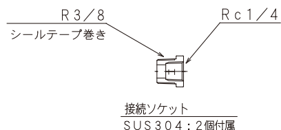
口径：1/4B サイズの構造
