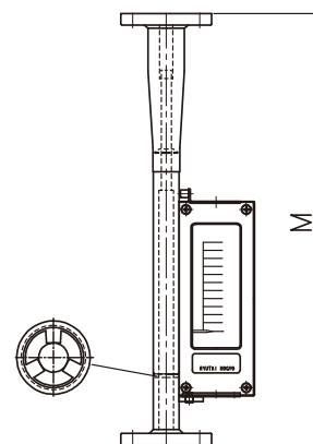
流れ方向記号：1 EMW 本体：80A以下
