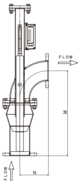
EMR102 標準形
