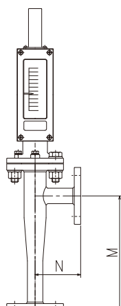
流れ方向記号：2
