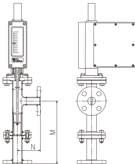
EMT 流れ方向記号：2
