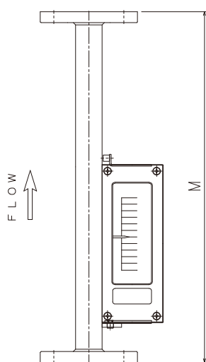
EMT 流れ方向記号：1
