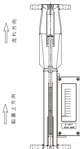
流れ方向 記号：1 取付方向
