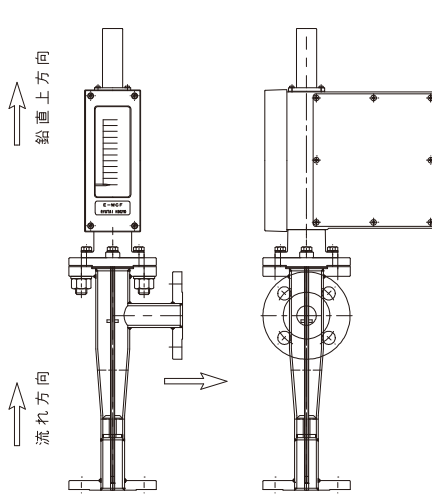
流れ方向 記号：2 取付方向
