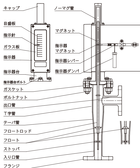
磁気追従式の構造例
