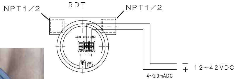
差圧伝送器 端子部
